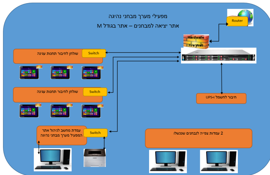
5.1.4. אתר בגודל M, להלן המחשה לשרטוט סכמתי של האתר:
