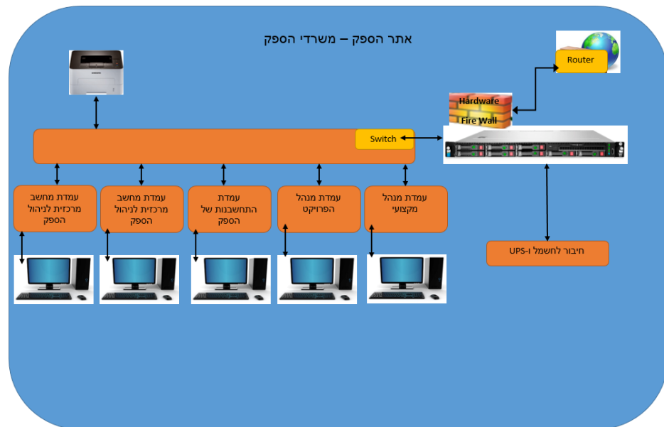
5.1.2. שרטוט סכמתי לאתר משרדי הספק:
